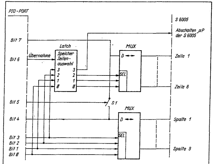
Bild 1 Prinzipschaltung
