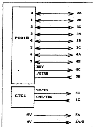
Bild 1 User-Port des KC-85/1
